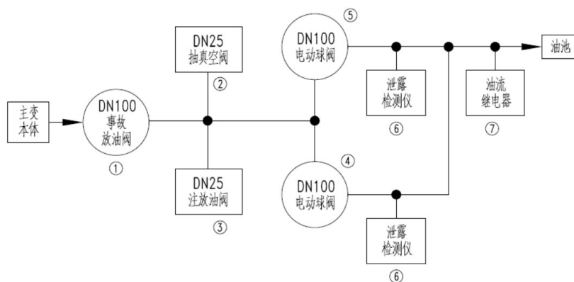
图 1 抽水蓄能电站主变压器应急排油系统设备配置图
