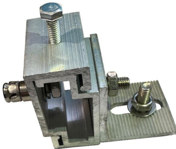
C 型子母式背栓挂件示意图
