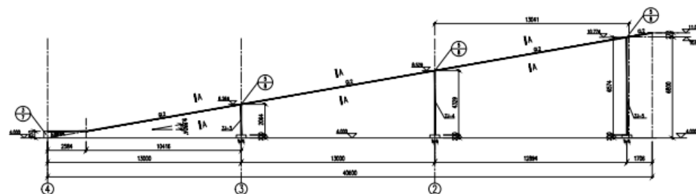
海缆运输桥架B轴结构立面图 1:100
