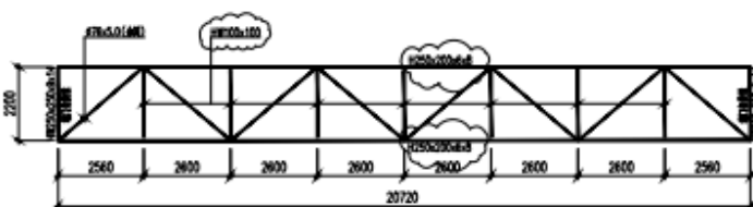
HJ-1 上弦支撑图 1:100
