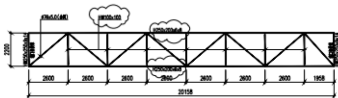
HJ-2 上弦支撑图 1:100
