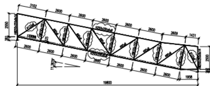
HJ-2 立面结构图 1:100
