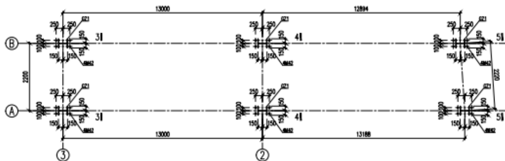
海缆运输桥梁支架柱平面布置图之二 1:50
