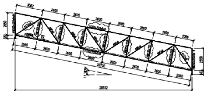
HJ-1 立面结构图 1:100
