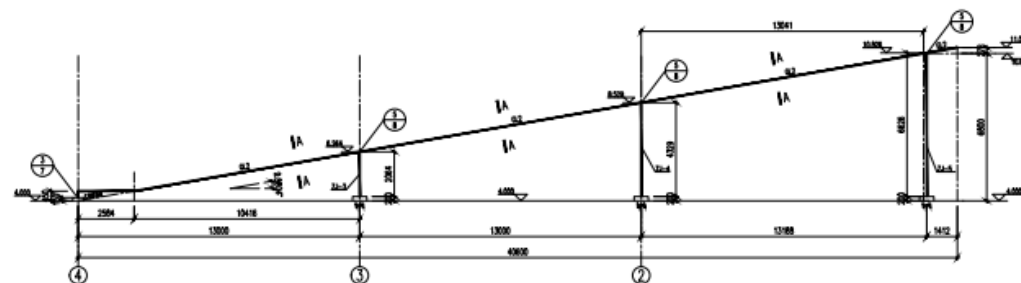
海缆运输桥架A轴结构立面图 1:100
